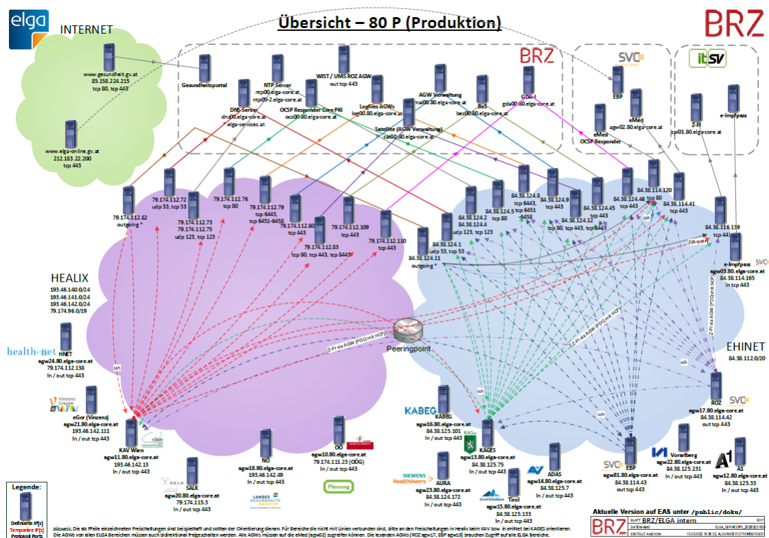
Abbildung 6: Topologie der Gesundheitsnetze
