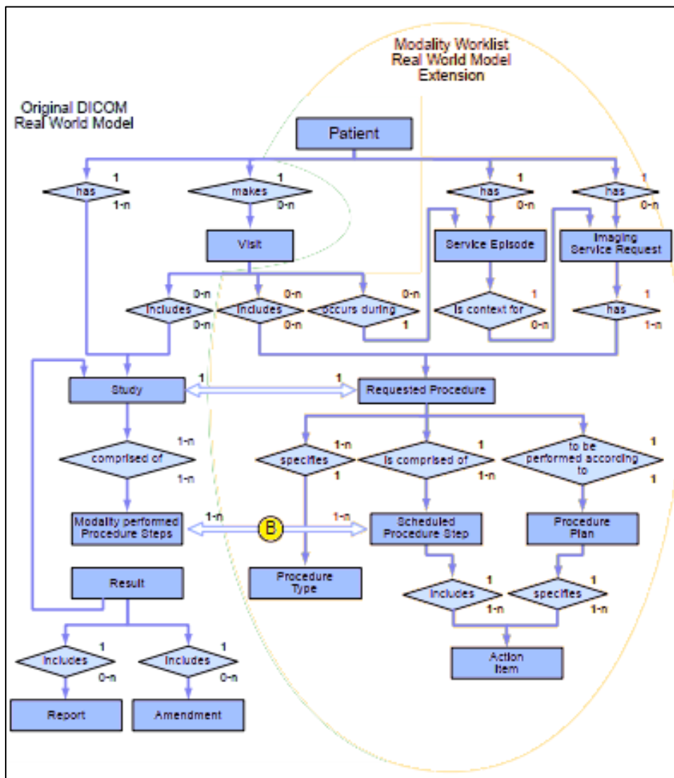
Abbildung 8: Datenmodell des Scheduled Workflows
