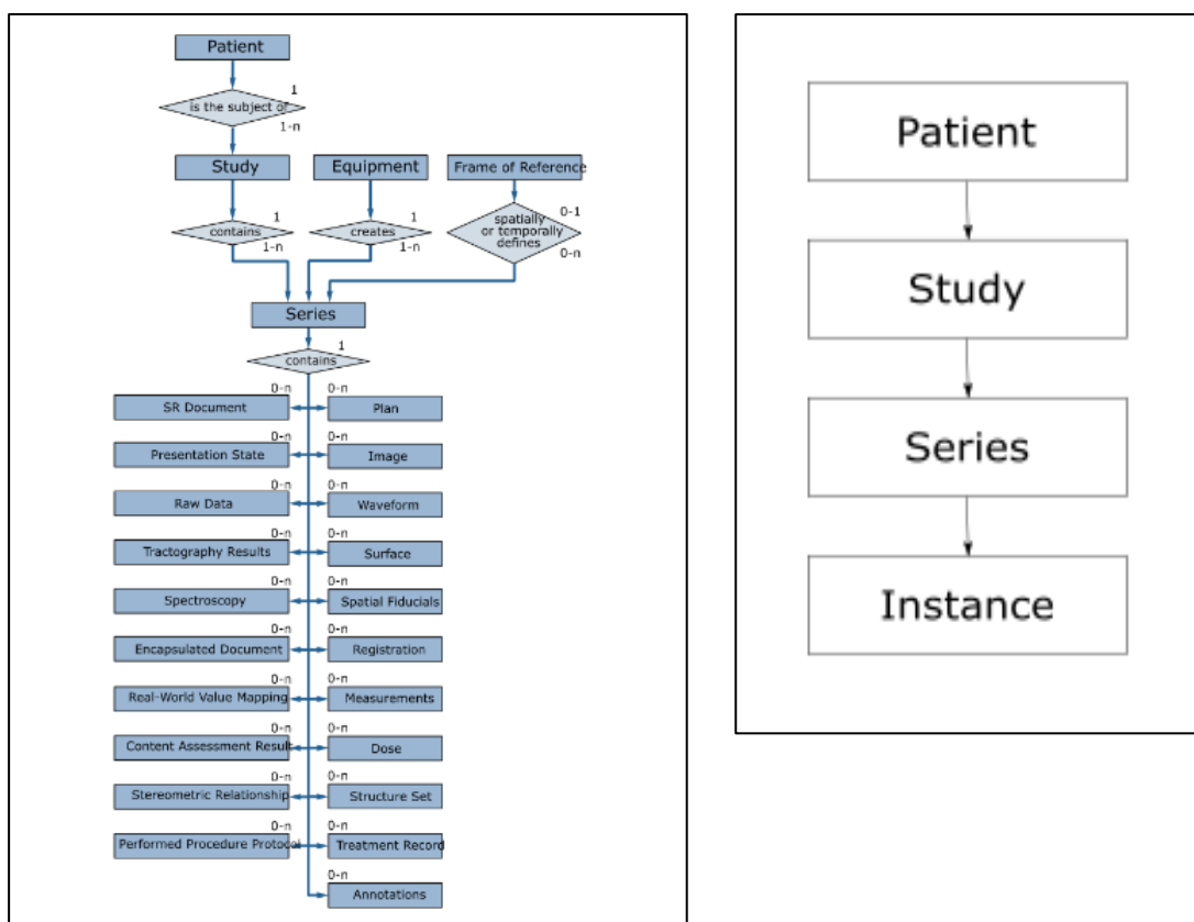
Abbildung 7: Datenmodell für DICOM Composite Information Objects
